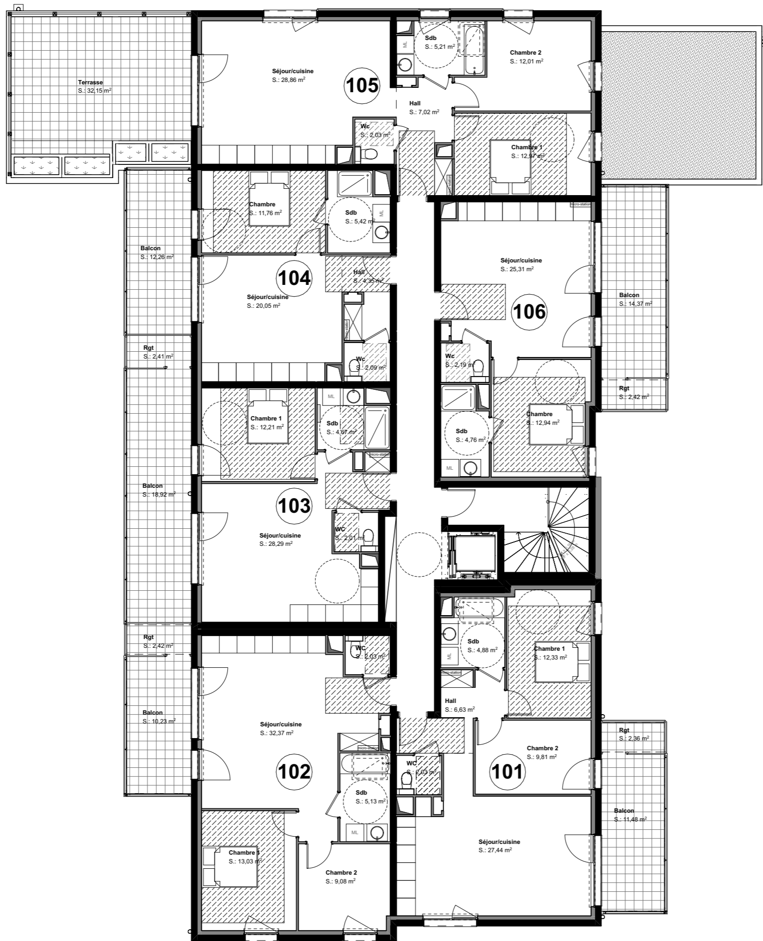
PLAN DU 1er ETAGE
