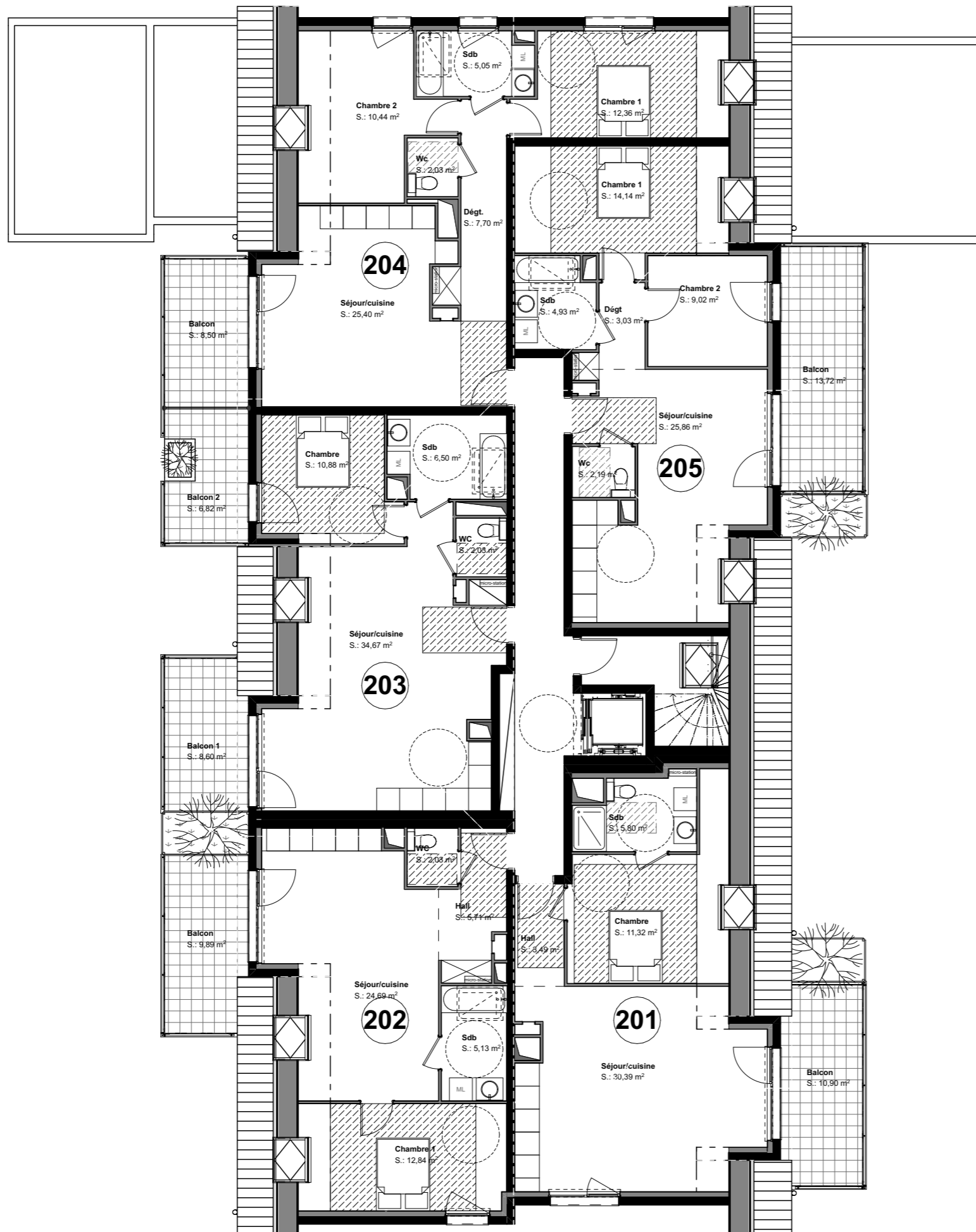
PLAN DES COMBLES
